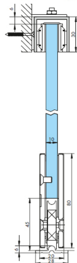
Настенный крепеж
